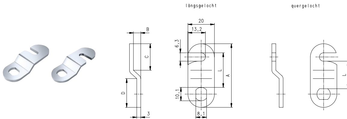
Hakenausnehmung links
