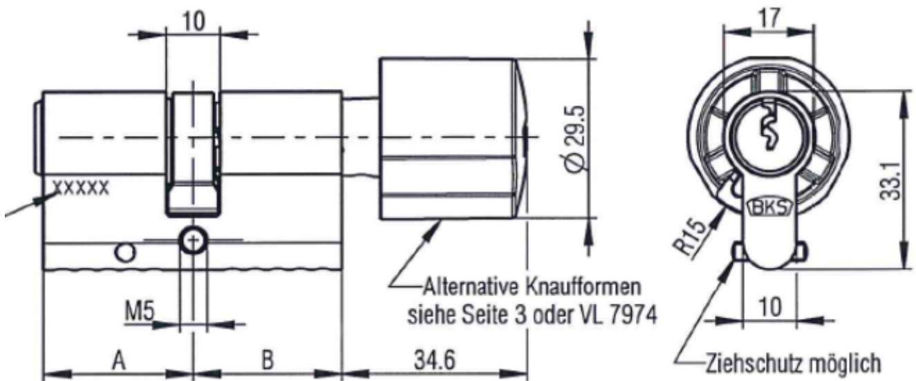
Knaufzylinder
