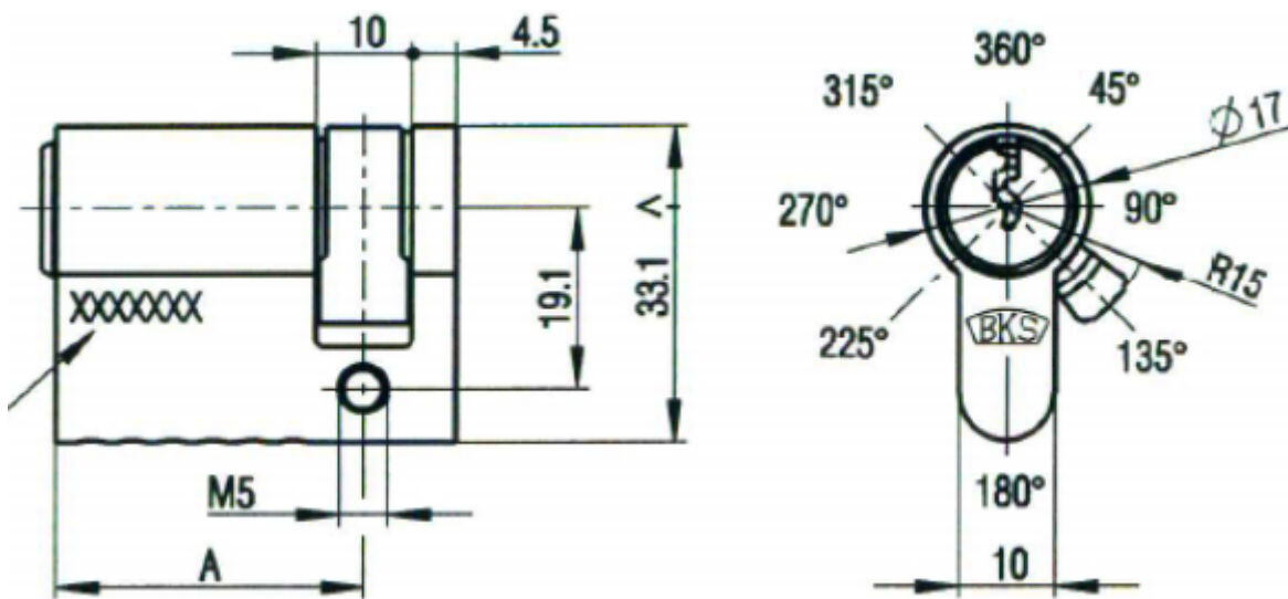
Halbzylinder
