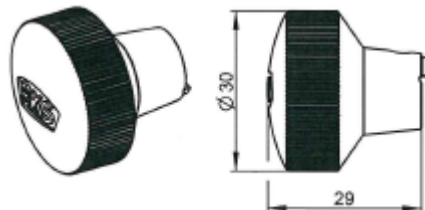
BKS-Rändelknauf
