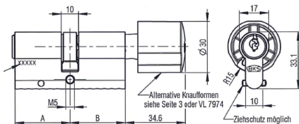
Knaufzylinder
