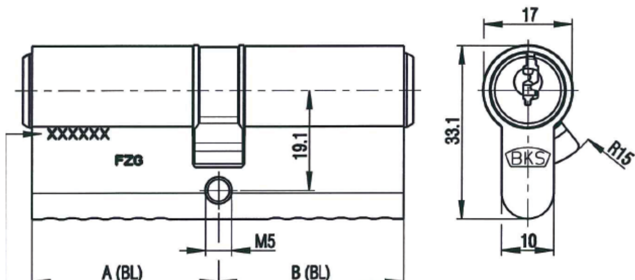
BKS-Designknauf
