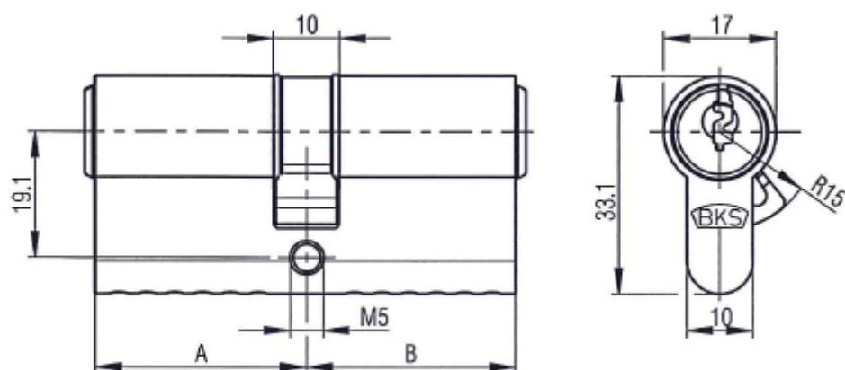
Doppelzylinder
