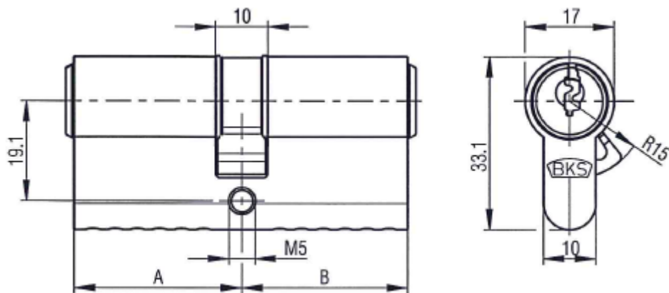
Doppelzylinder
