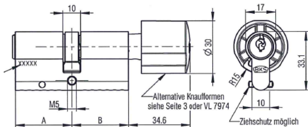
Knaufzylinder
