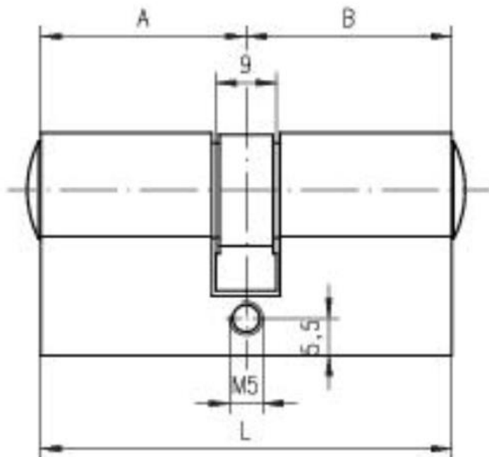
Doppelzylinder
