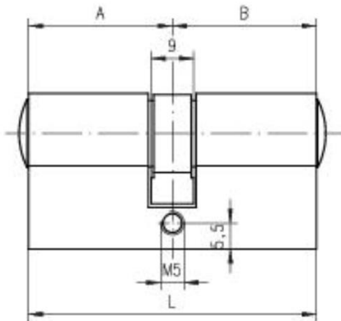
Hebelzylinder
