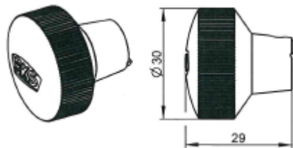
BKS-Rändelknauf
